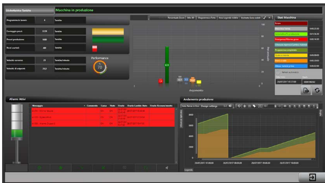
2. Stato della macchina etichettatrice realizzata con Movicon.NEXt
