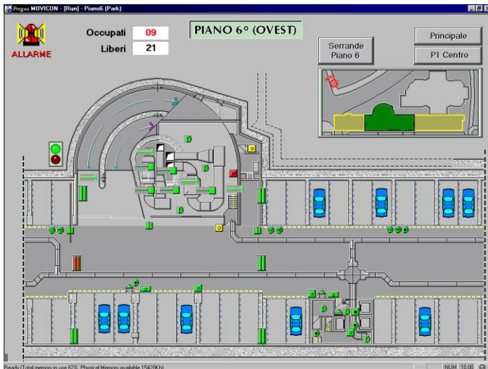
Uno dei sinottici visibili dalla postazione di controllo dell'operatore del parcheggio.
